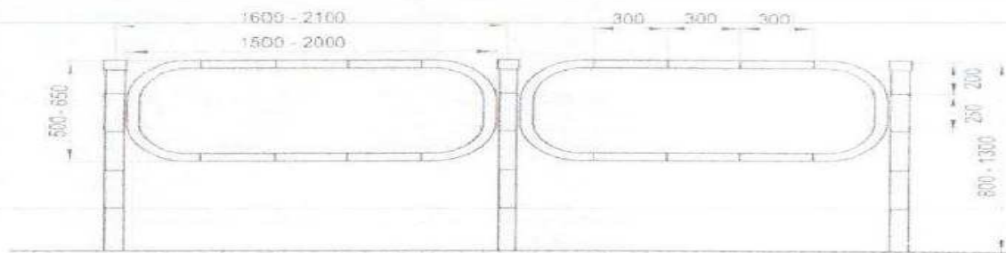
Rysunek 4 - Sposób zamocowania balustrad w podłożu
